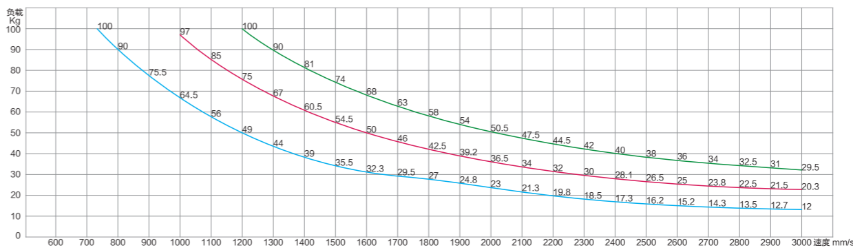
电机加速度和减速度时间各0.1S, 停顿时间0.2S 电机加速度和减速度时间各0.2S, 停顿时间0.2S 电机加速度和减速度时间各0.3S, 停顿时间0.3S 短行程、推荐使用三角形速度模式(无匀速), 长行程推荐梯形速度模式
